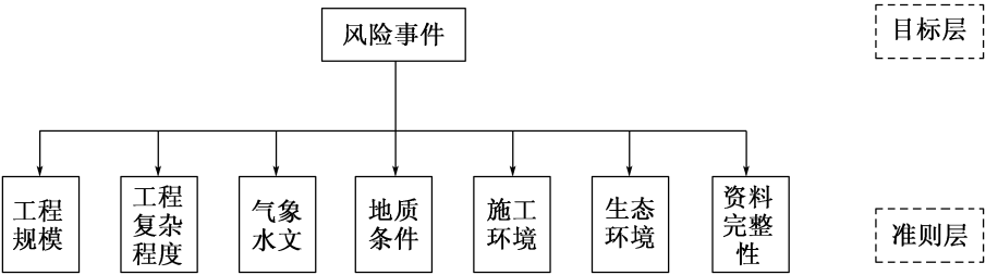
图 B.1 递阶层次结构
